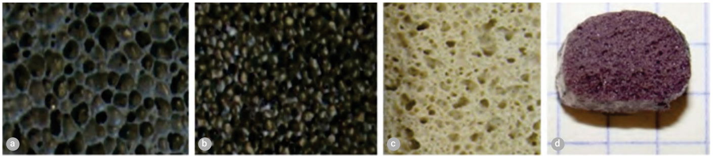
5. Mousses issues du mélange de verre avec différents agents porogènes. (a) Carbure de silicium SiC. (b) Carbone (graphite). (c) Nitrure d'aluminium AlN. (d) C + MnO 2 .
